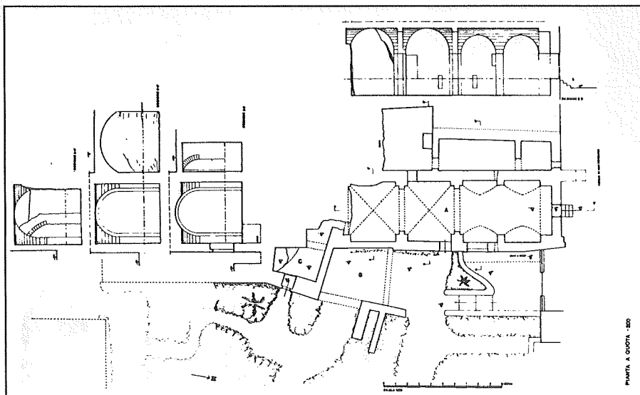
Fig. 29 - Palermo, Complesso di San Giovanni degli Eremiti: pianta del pian terreno dell'edificio adiacente alla corsia Nord del chiostro, scala 1:50 (rilievo di T. Torregrossa 1986).
