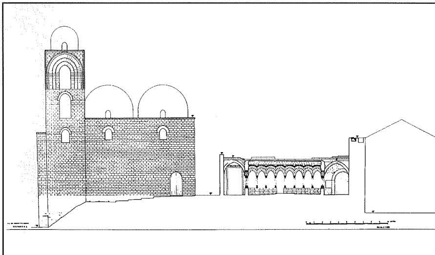
Fig. 12 - Palermo, Chiesa e chiostro di San Giovanni degli Eremiti: sezione scala 1:50 (rilievo di T. Torregrossa 1986).
