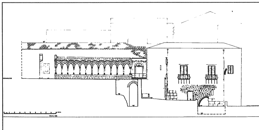
Fig. 30 - Palermo Complesso di San Giovanni degli Eremiti: sezione del chiostro e prospetto orientale dell'edificio adiacente sul lato Nord, scala 1:50 (rilievo di T. Torregrossa 1986).
