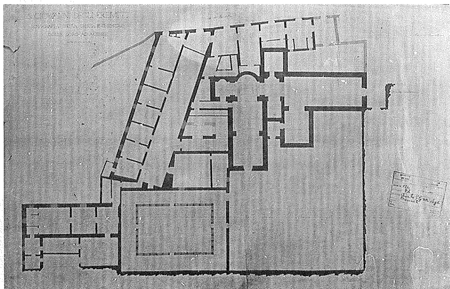
Fig. 5 - Palermo, Complesso di San Giovanni degli eremiti: planimetria antecedente alle demolizioni del 1875, scala 1:100 (Archivio della Soprintendenza ai BB.CC.AA. di Palermo).
