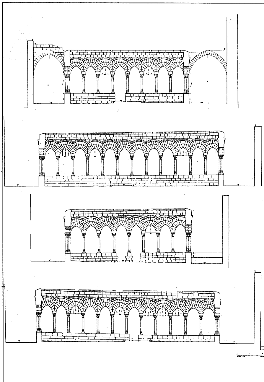
Fig. 13 - Palermo, Chiostro di San Giovanni degli Eremiti: sezioni, scala 1:20 - rilievi di T. Torregrossa, 1986.
