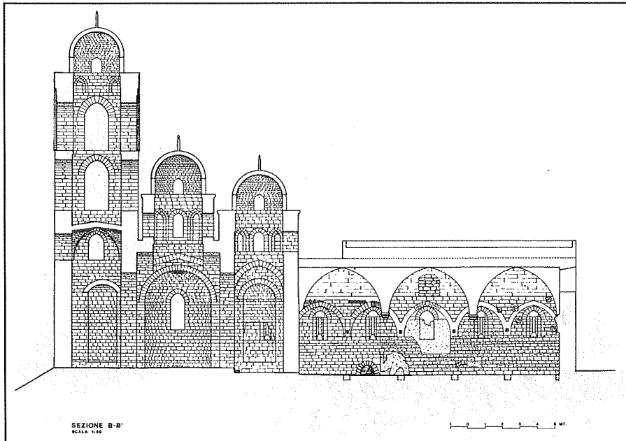
Fig. 7 - Palermo, Chiesa di San Giovanni degli Eremiti: sezione trasversale, scala 1:50 (rilievo di A. Daidone 1986).
