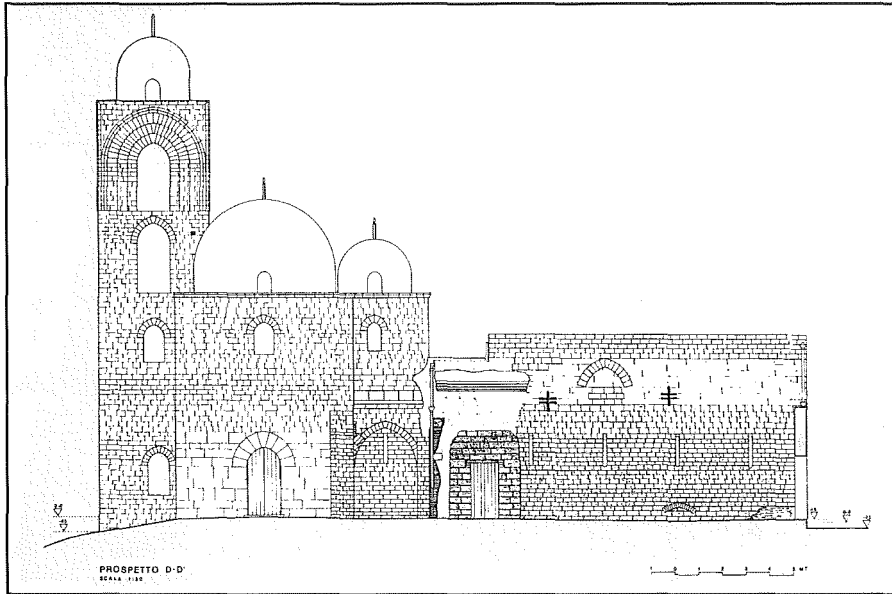
Fig. 19 - Palermo, Chiesa di San Giovanni degli Eremiti: prospetto principale della chiesa e della sala adiacente, scala 1:50 (rilievo di A. Daidone 1986).
