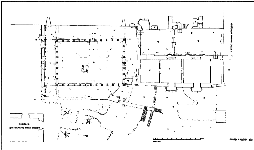
Fig. 11 - Palermo, Chiostro di San Giovanni degli Eremiti: planimetria, scala 1:50 (rilievo di T. Torregrossa 1986).
