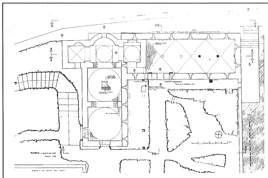
Fig. 6 - Palermo, Chiesa di San Giovanni degli Eremiti: pianta, scala 1:50 (rilievo di A. Daidone 1986).
